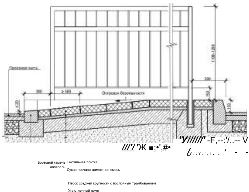
Илл 5.4.1. ПРИНЦИПАЛЬНАЯ СХЕМА УСТРОЙСТВА ОСТРОВКА БЕЗОПАСНОСТИ С ОГРАЖДЕНИЯМИ С ПОКРЫТИЕМ ИЗ БЕТОННОЙ ПЛИТКИ / ПЛИТКИ ИЗ НАТУРАЛЬНОГО КАМНЯ С ПРОЕЗЖЕЙ ЧАСТЬЮ (СЕЧЕНИЕ).
