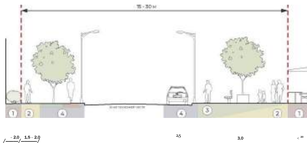
ИЛЛ. 5.4. ПРОФИЛЬ УЛИЦЫ В ОБЩЕСТВЕННО-ДЕЛОВЫХ И ТОРГОВЫХ ЗОНАХ
