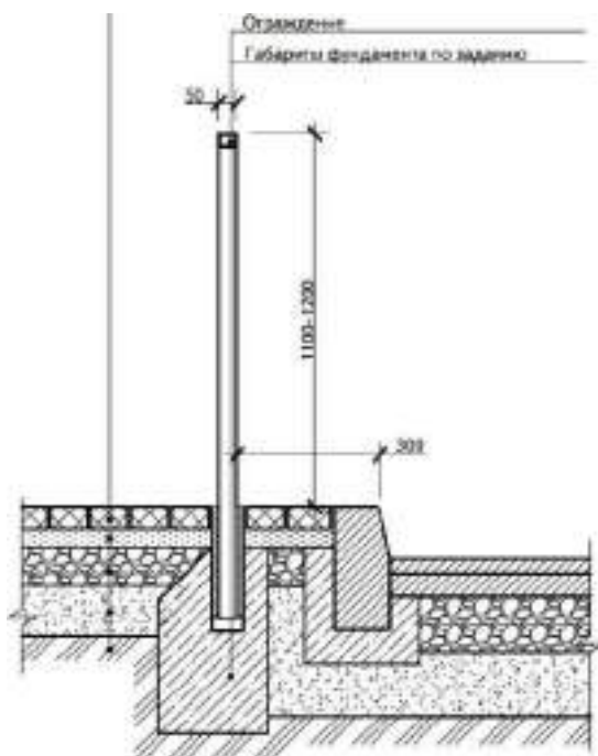
Илл. 5.4.2. ПРИНЦИПИАЛЬНАЯ СХЕМА МОНТАЖА ПЕШЕХОДНОГО ОГРАЖДЕНИЯ
