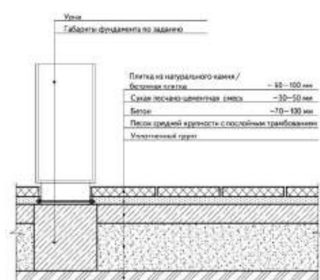
Илл. 5.2.1. ПРИНЦИПИАЛЬНАЯ СХЕМА МОНТАЖА УРНЫ В МОЩЕНИЕ
