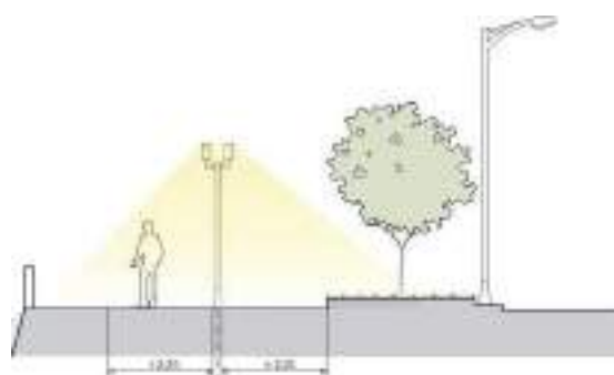
ИЛЛ. 1.15 ОСЕВАЯ СХЕМА РАСПОЛОЖЕНИЯ ОПОР ОСВЕЩЕНИЯ
