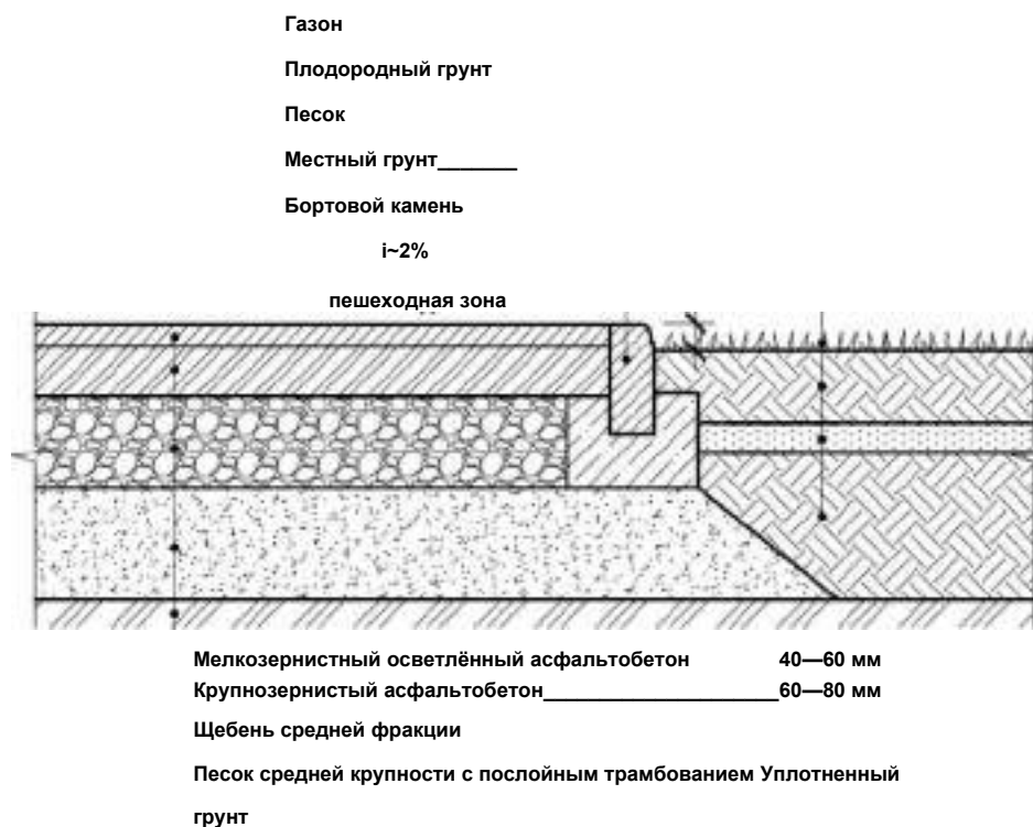
Илл. 1.2.2. ПРИНЦИПИАЛЬНАЯ СХЕМА СОПРЯЖЕНИЯ ПЕШЕ
