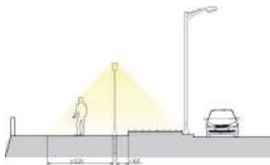
ИЛЛ. 1.14 ОДНОСТОРОННЯЯ СХЕМА РАСПОЛОЖЕНИЯ ОПОР ОСВЕЩЕНИЯ
