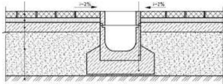
Илл. 1.2.13. ПРИНЦИПАЛЬНАЯ СХЕМА УСТРОЙСТВА ЛИВНЕВОГО ВОДООТВОДА ПЕРПЕНДИКУЛЯРНО ПЕШЕХОДНОЙ ЗОНЕ
