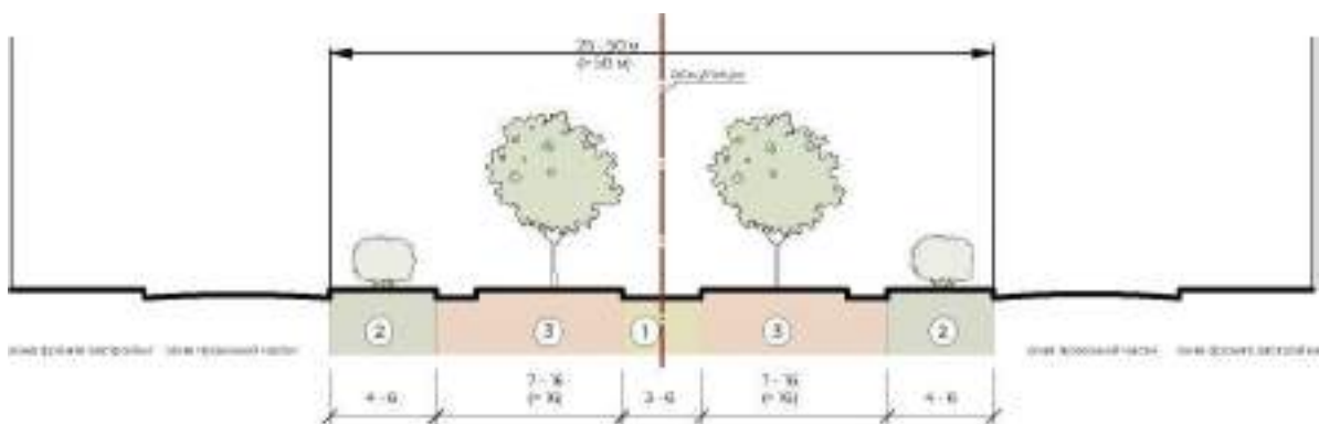
Бульвар по оси улицы Вариант 2
