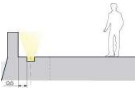
Светильник, встроенный в покрытие береговой зоны
