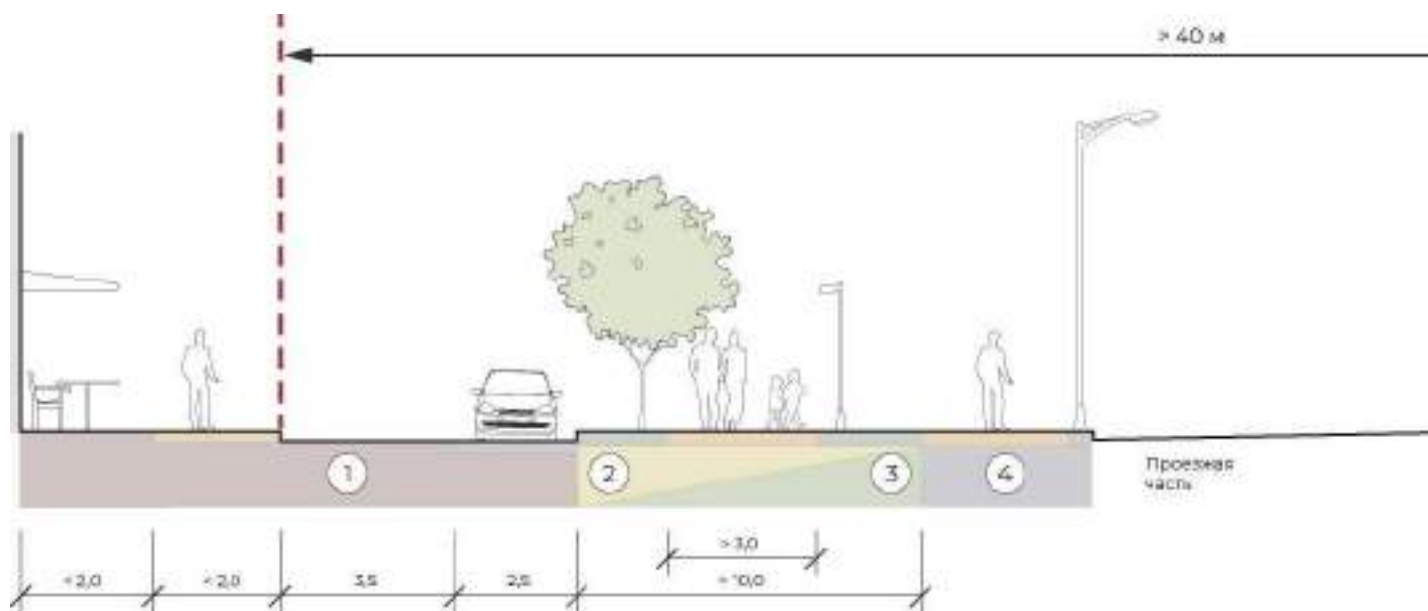
Илл. 5.2. ПРОФИЛЬ МАГИСТРАЛЬНОЙ УЛИЦЫ ОБЩЕГОРОДСКОГО И РАЙОННОГО ЗНАЧЕНИЯ
