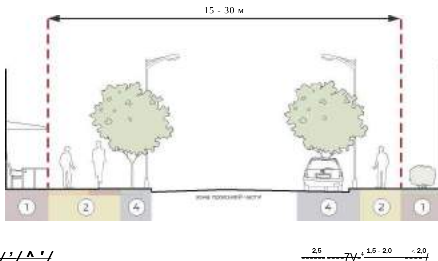
Илл. 5.3. ПРОФИЛЬ УЛИЦЫ В ЖИЛОЙ ЗАСТРОЙКЕ
