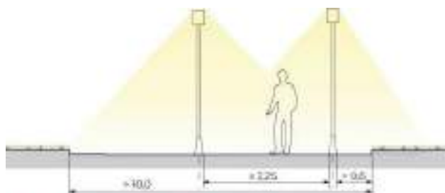
ИЛЛ. 5.13. ДВУХРЯДНАЯ ПРЯМОУГОЛЬНАЯ СХЕМА РАСПОЛОЖЕНИЯ ОПОР ОСВЕЩЕНИЯ
