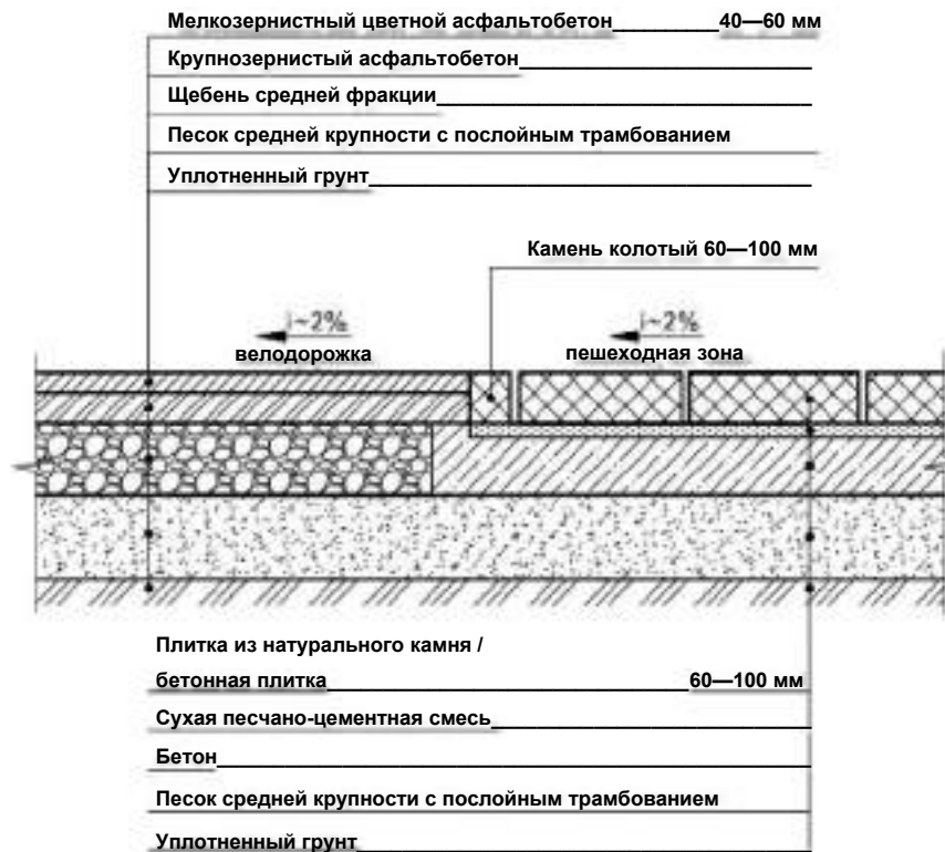
Илл. 1.2.8. ПРИНЦИПИАЛЬНАЯ СХЕМА СОПРЯЖЕНИЯ ПЕШЕ ХОДНОЙ ЗОНЫ ИЗ БЕТОННОЙ ПЛИТКИ (ПЛИТКИ ИЗ
