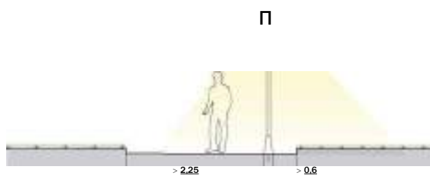
ИЛЛ. 5.11. ОДНОСТОРОННЯЯ СХЕМА РАСПОЛОЖЕНИЯ ОПОР ОСВЕЩЕНИЯ
