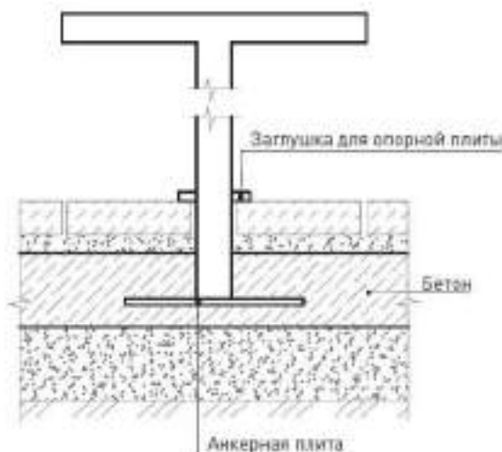
Илл. 3.3.2. ПРИНЦИПАЛЬНАЯ СХЕМА УСТРОЙСТВА СТОЛА ПРИ ПОМОЩИ АНКЕРНОЙ ПЛИТЫ
