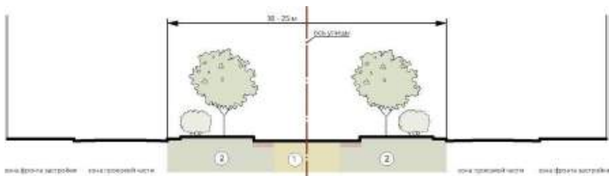
Бульвар по оси улицы Вариант 1
