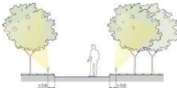
Илл.6.16. ОСВЕЩЕНИЕ ЗЕЛЕННЫХ НАСАЖДЕНИЙ
