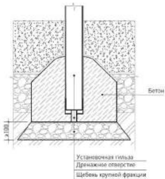
ИЛЛ. 3.2.2. СХЕМА МОНТАЖА СПОРТИВНОГО ОБОРУДОВАНИЯ В ПОКРЫТИЕ ИЗ НАСЫПНОГО
