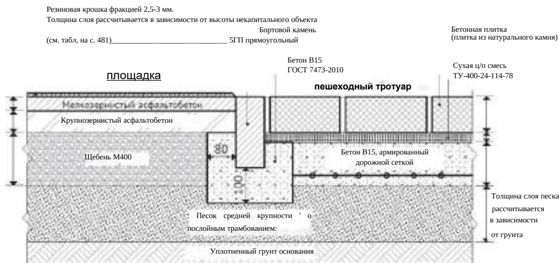
Илл. 3.1.10. ПРИНЦИПАЛЬНАЯ СХЕМА УСТРОЙСТВА СОПРЯЖЕНИЯ ПОКРЫТИЯ ДЕТСКОЙ ПЛОЩАДКИ С ПОКРЫТИЕМ ИЗ БЕТОННОЙ ПЛИТКИ (РЕШЕНИЕ УТОЧНЯЕТСЯ ИНДИВИДУАЛЬНО В ПРОЕКТЕ В ЗАВИСИМОСТИ ОТ
