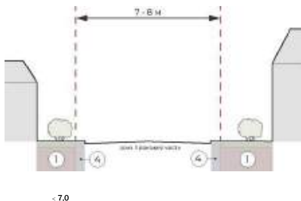
Илл. 5.8. ПРОФИЛЬ МЕСТНОЙ УЛИЦЫ СЕЛЬСКИХ ПОСЕЛЕНИЙ
