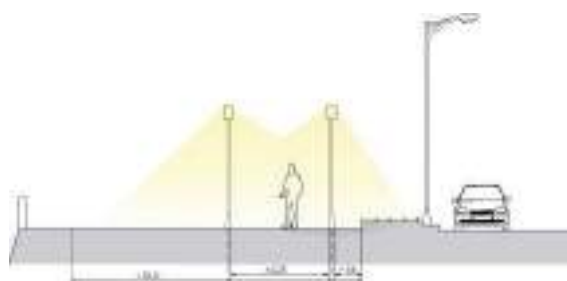
ИЛЛ. 1.16 ДВУХЯРДНАЯ ПРЯМОУГОЛЬНАЯ СХЕМА РАСПОЛОЖЕНИЯ ОПОР ОСВЕЩЕНИЯ
