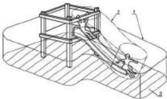
Илл. 3.1.1. Зоны игрового оборудования: 1 - зона падения; 2 ~ зона безопасности; 3 ~ зона приземления (ГОСТ Р 52169)
