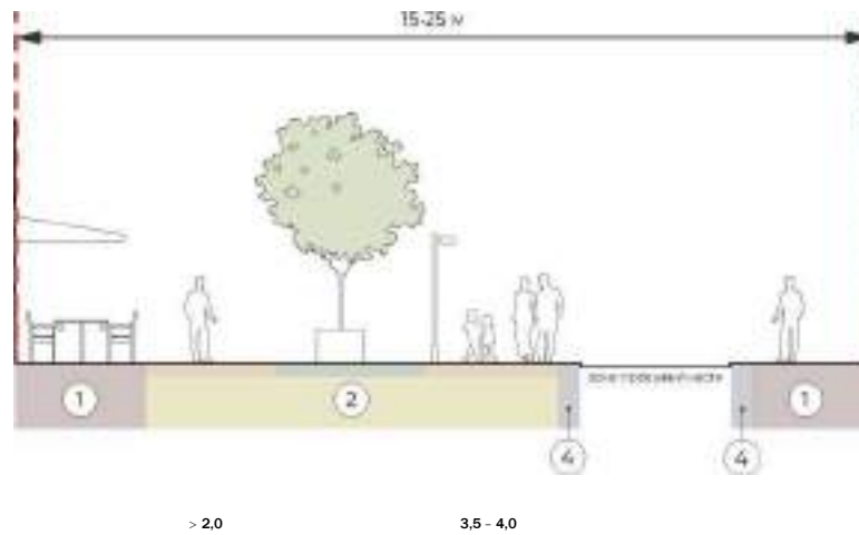
Илл. 5.6. ПРОФИЛЬ УЛИЦЫ С ЧАСТИЧНЫМ ОГРАНИЧЕНИЕМ АВТОМОБИЛЬНОГО ДВИЖЕНИЯ
