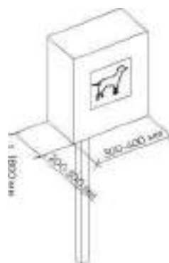
Урна для отходов жизнедеятельности животных
