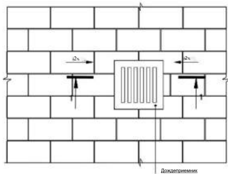
Илл. 1.2.14. ПРИНЦИПАЛЬНАЯ СХЕМА УСТРОЙСТВА ДОЖДЕ
