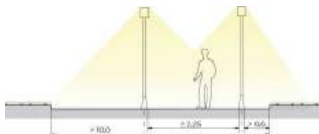
Илл. 4.1.5. ДВУХРЯДНАЯ ПРЯМОУГОЛЬНАЯ СХЕМА РАСПОЛОЖЕНИЯ ОПОР ОСВЕЩЕНИЯ
